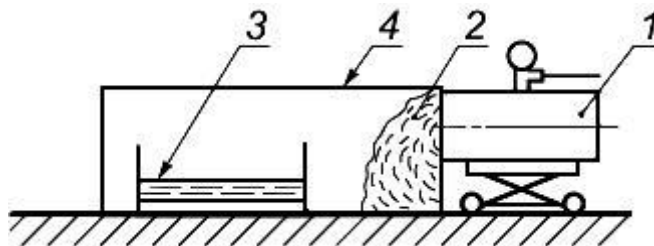
Рисунок 9 - Схема установки
