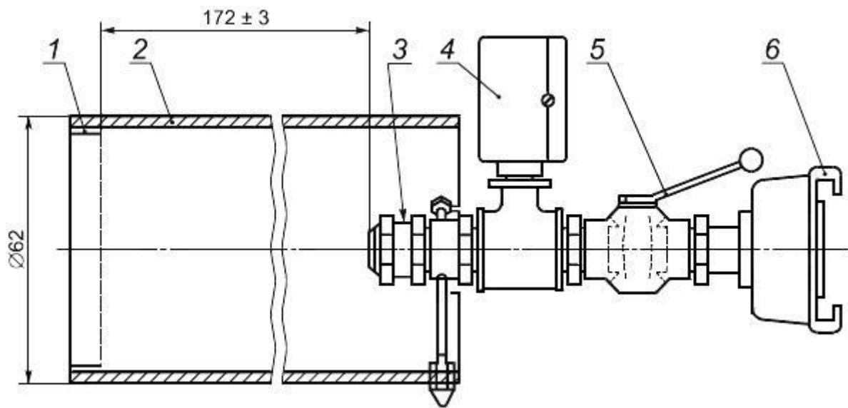
Рисунок 8 - Пожарный ствол пены средней кратности
