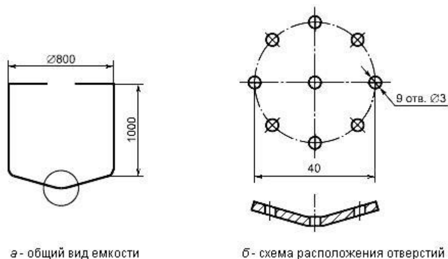
Рисунок 5 - Емкость для сбора пены
