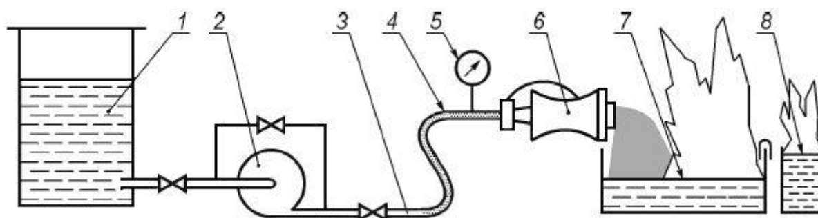
Рисунок 7 - Схема установки для тушения пеной средней кратности
